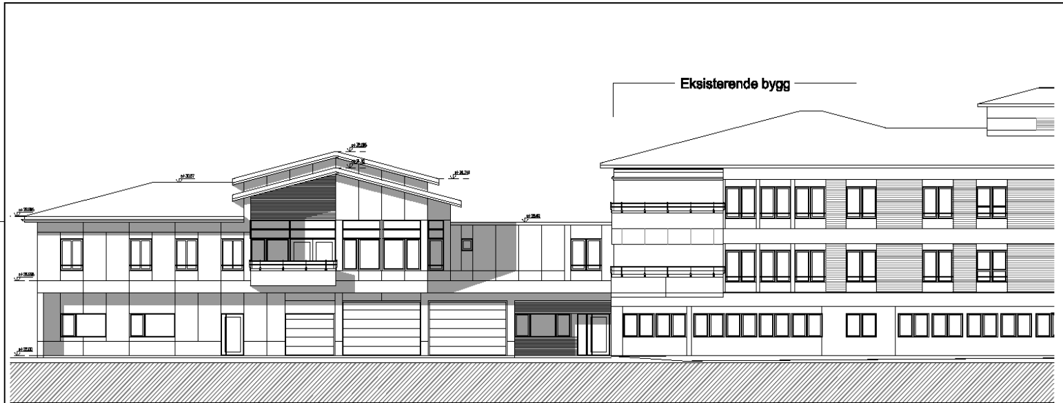
FASADE SYD
